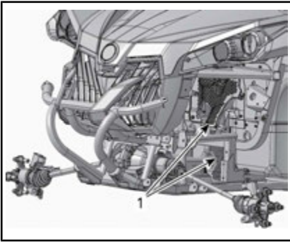
TYPIQUE - AVANT DU VÉHICULE - COMPOSANTS RETIRÉS POUR PLUS DE CLARTÉ
