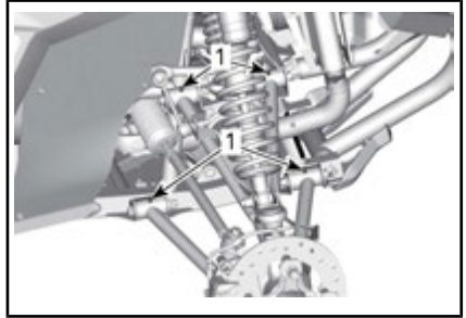
SUSPENSIÓN DELANTERA - TÍPICO
