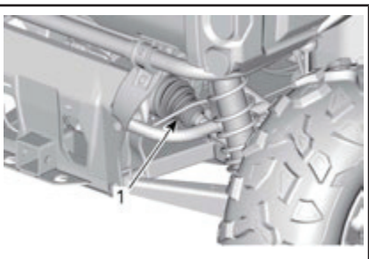
ACHTERKANT VOERTUIG
