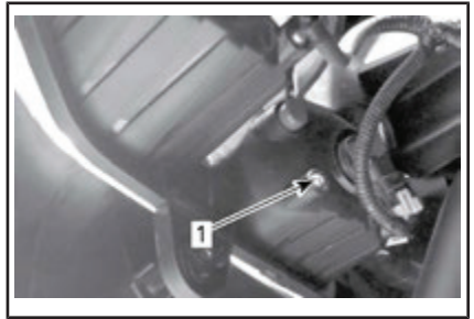
1. Afstelschroef
