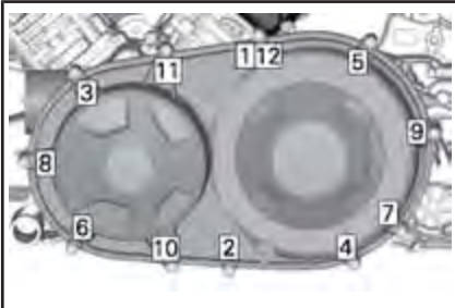
CVT:N (PORTAATON VOIMANSIIRTO) KANNEN KIRISTÄMISJÄRJESTYS
