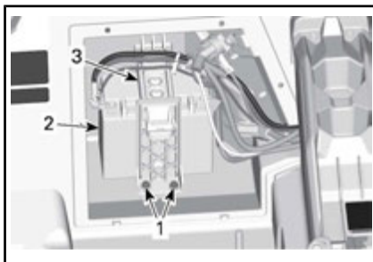
1. Tornillos de sujeción del portabaterías 2. Batería 3. Portabaterías
