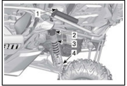
TÍPICO - MODELOS MAVERICK X3 X RS - SUSPENSIÓN TRASERA
