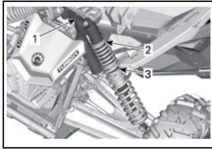
TÍPICO - MODELOS MAVERICK X3 - SUSPENSIÓN DELANTERA
