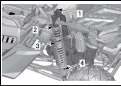
TÍPICO - MODELOS MAVERICK X3 X DS - SUSPENSIÓN TRASERA
