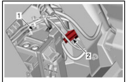
1. Batería 2. Fusible del DPS
