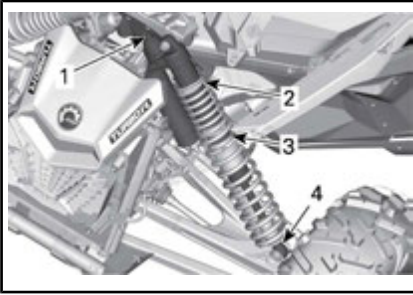
TÍPICO - MODELOS MAVERICK X3 X DS Y X RS - SUSPENSIÓN DELANTERA
