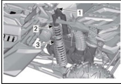
TÍPICO - MODELOS MAVERICK X3 MAX - SUSPENSIÓN TRASERA
