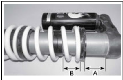
TÍPICO - AJUSTE DE LA SUPERPOSICIÓN - AMORTIGUADOR TRASERO
