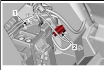
1. Batería 2. Fusible de la DPS
