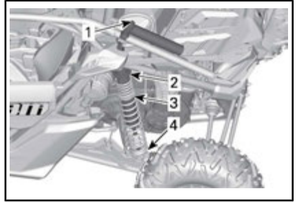
TÍPICO - MODELOS MAVERICK X3 MAX X rsRS - SUSPENSIÓN TRASERA
