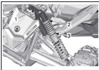
典型示例 - MAVERICK X3 MAX 车型 - 前悬架
