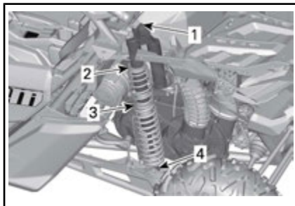
典型示例 - MAVERICK X3 MAX X DS 车型 - 后悬架
