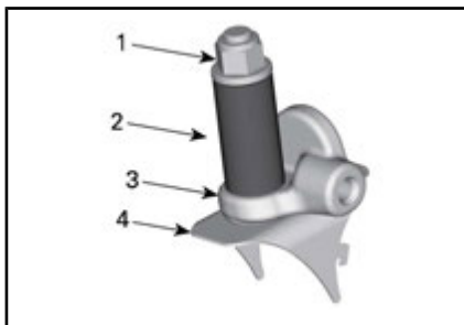
低位后锚点
