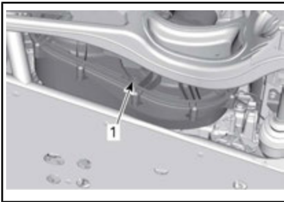
1. CVT 排水口
