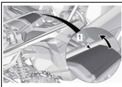
1. 前检修盖
