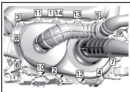
TYPISCH - ANZUGSREIHENFOLGE DER CVT-ABDECKUNG
