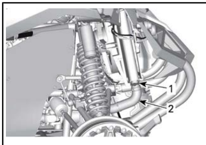
1. Zu notierende Position der Schlauchschelle
