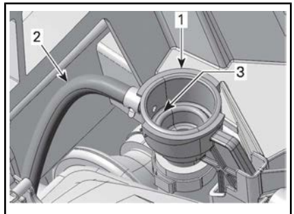
1. Adapter zum Auffüllen des Kühlsystems 2. Schlauch des Ausgleichsbehälters 3. Kühlsystem befüllt (Sitz der Druckkappe)
