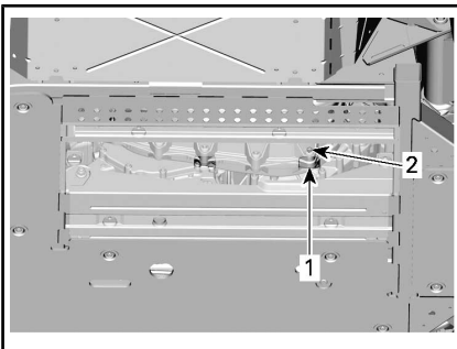
SCHUTZPLATTE ENTFERNT - TYPISCH
