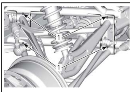
HINTERE AUFHÄNGUNG - TYPISCH
