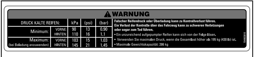
HINWEISSCHILD 7
