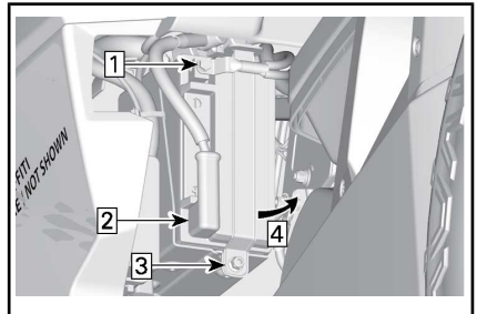
1. ZWARTE (-) kabel
