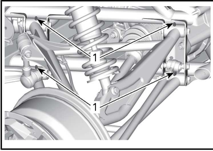
TYPISCH - ACHTERWIELOPHANGING
