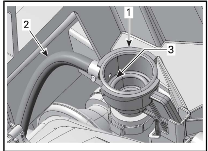
1. Adapter bijvullen koelsysteem 2. Slang expansievat 3. Koelsysteem volledig gevuld (tot zitting drukdop)
