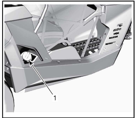
1. Dop brandstoftank
