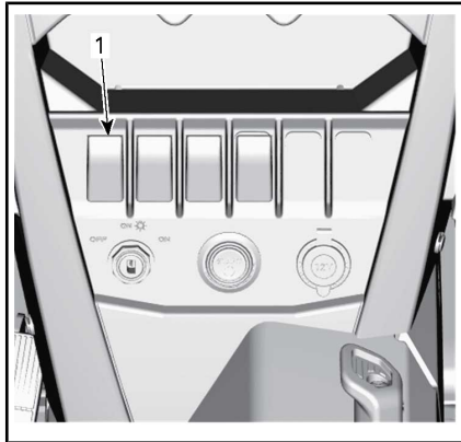
1. Knipperlichtschakelaar
