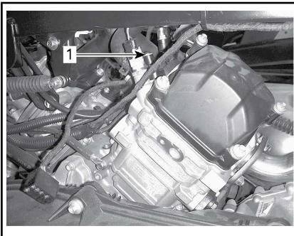
1. Ontluchtingsschroef cilinder achteraan 2. Verwijder de drukdop.
