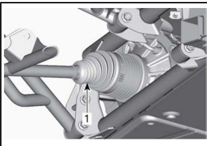
TYYPILLINEN – AJONEUVON TAKAOSA (OSAT POISTETTU SELVYYDEN VUOKSI)
