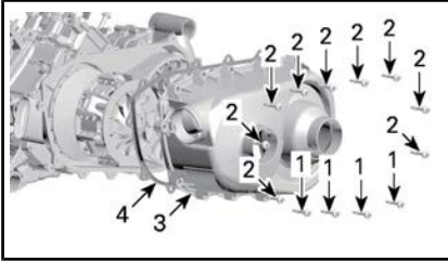
CVT:N (PORTAATON VOIMANSIIRTO) KANNEN KIRISTÄMISJÄRJESTYS
