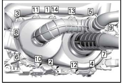
CVT:N (PORTAATON VOIMANSIIRTO) KANNEN KIRISTÄMISJÄRJESTYS
