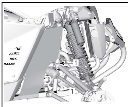
TYPISCH - VORDERRADAUFHÄNGUNG
