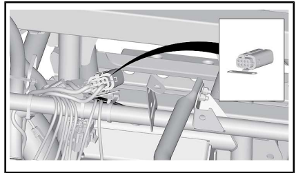
DRITTER SICHERUNGSKASTEN - HINTER OBERER KONSOLE
