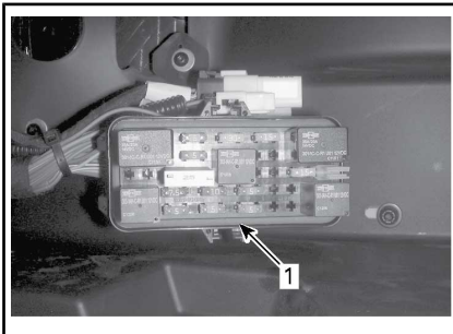
1. Hauptsicherungskasten
