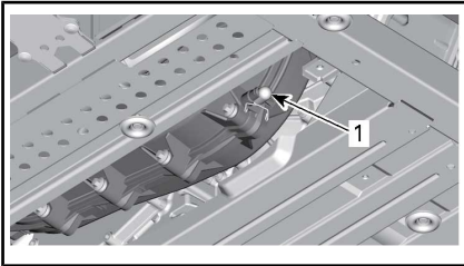
1. CVT-Entleerung
