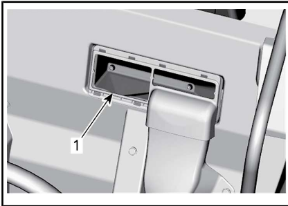
1. Hinterer CVT-Luftfilter
