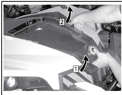
Schritt 1: Heben Sie die Vorderseite der Wartungsabdeckung weiter an
