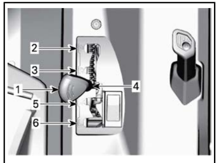
1. Schalthebel 2. Parken 3. Rückwärts 4. Neutral 5. Bereich für hohe Geschwindigkeit (vorwärts) 6. Bereich für niedrige Geschwindigkeit (vorwärts)
