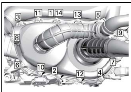
Normal - ANZUGSABFOLGE CVT-ABDECKUNG
