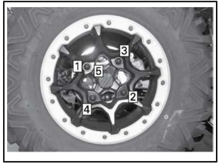
REIHENFOLGE BEIM ANZIEHEN
