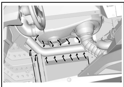
TYPISCH - TEILE AUS GRÜNDEN DER ÜBERSICHTLICHKEIT ENTFERNT
