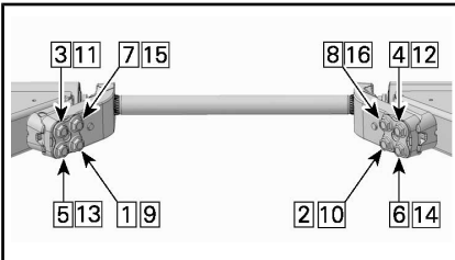
SEQUENZA DI SERRAGGIO DELLA BARRA DI STABILIZZAZIONE
