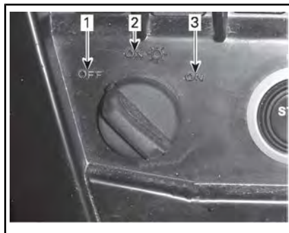
POSIZIONE DELL'INTERRUTTORE DI ACCENSIONE
