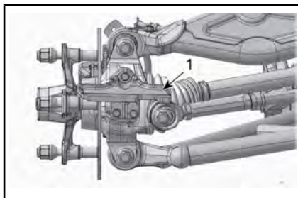
RUOTA RIMOSSA PER CHIAREZZA
