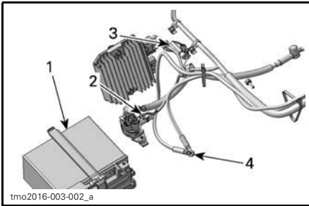
TYPIQUE - ILLUSTRATION À TITRE INDICATIF
