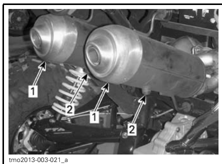
1. Silencieux 2. Bouchons de purge
