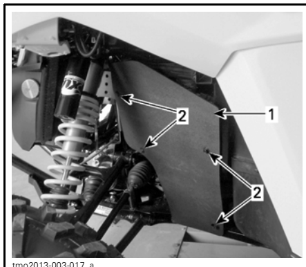
ACCÈS AU BOUCHON DE VIDANGE DEPUIS LE CÔTÉ GAUCHE DU VÉHICULE
