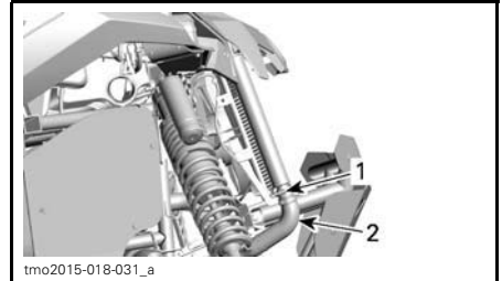
1. Position du collier de serrage à noter 2. Boyau inférieur de radiateur à retirer
