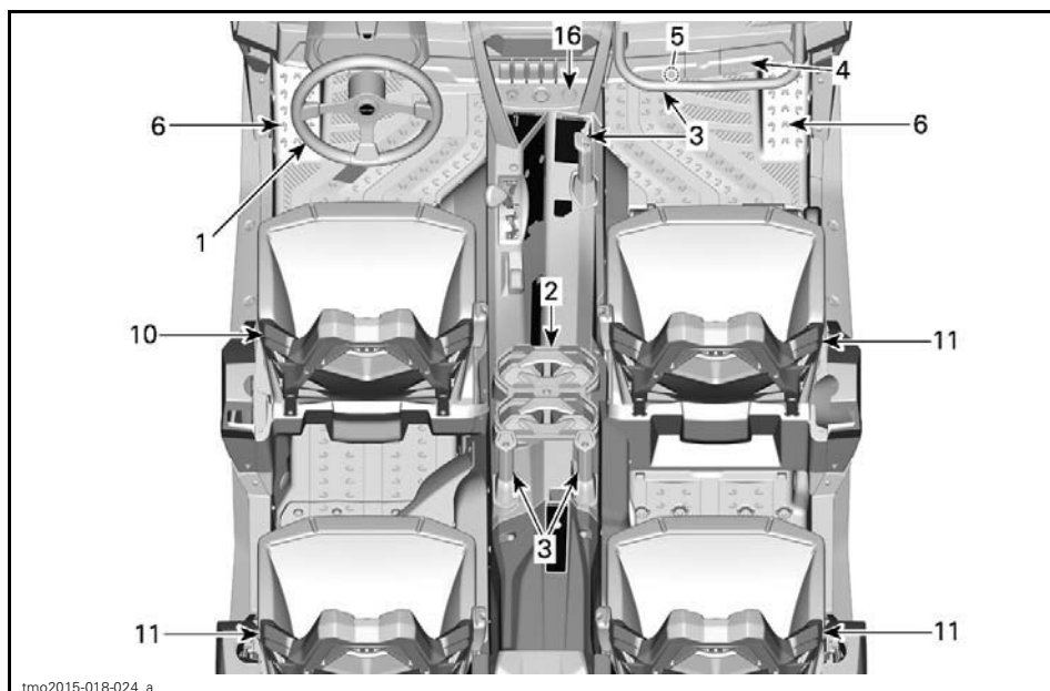
MODÈLE TURBOCOMPRESSÉ
