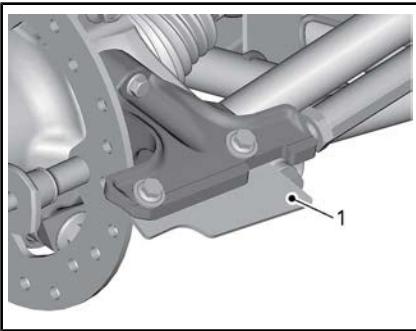
1. Pyöräraapan jatke
