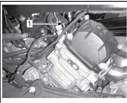
1. Takasynterinin ilmausruuvi
