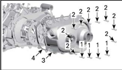
CVT:N (PORTAATON VOIMANSIIRTO) KANNEN KIRISTÄMISJÄRJESTYS
