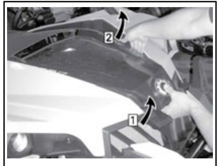
Etapa 1: Mantenga levantada la parte frontal de la tapa de servicio
