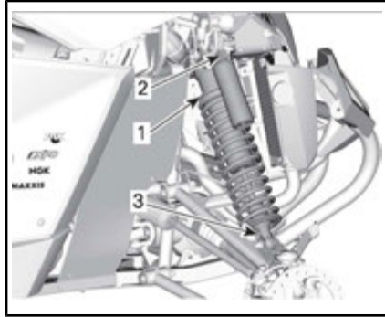
SUSPENSIÓN DELANTERA - TODOS LOS MODELOS EXCEPTO X xc
