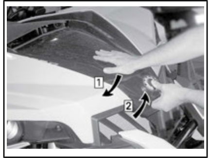
Etapa 1: Presione la tapa de servicio hacia abajo y MANTÉNGALA ASÍ
