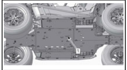
1. Acesso ao bujão de drenagem do sistema de arrefecimento
