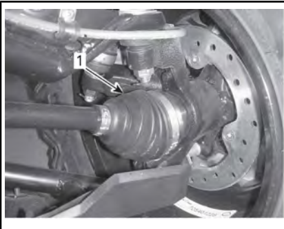
VOORZIJDE VOERTUIG
