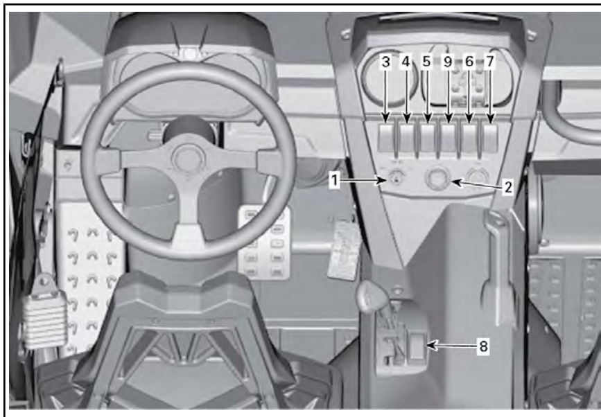
TÍPICO: MANDOS SECUNDARIOS
