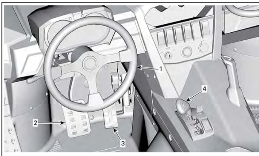
CONFIGURAZIONE TIPICA
