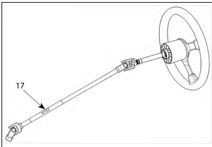
CONFIGURAZIONE TIPICA
