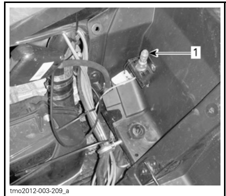
1. Aansluiting compressor
