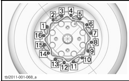
AANDRAAI VOLGORDE
