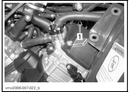
1. Hose pincher
