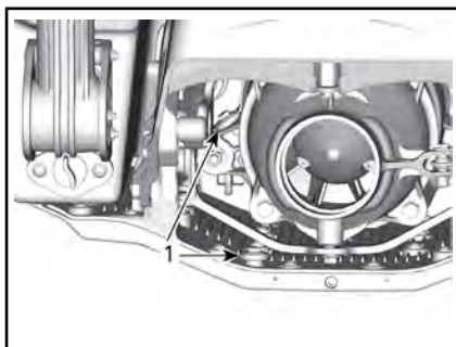
1. Anodes sacrificielles
