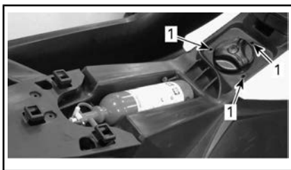
1. Винты
