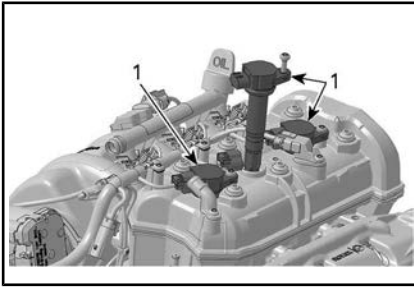
1. Катушки зажигания
