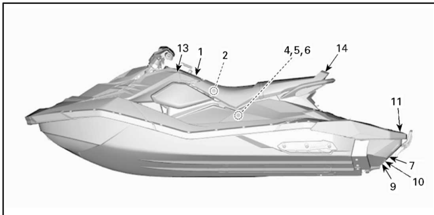
典型示例 - 三人型 - 配备 iBR 和便利包
