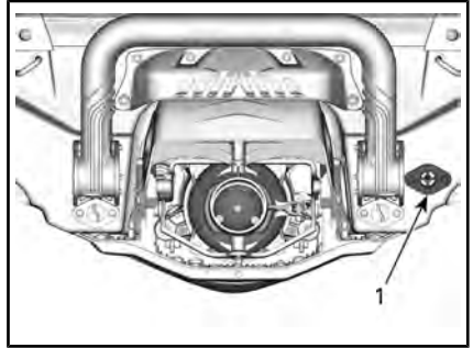
1. Spolanslutning
