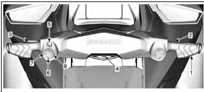
TYPISK- 2 KNAPPSATSER
