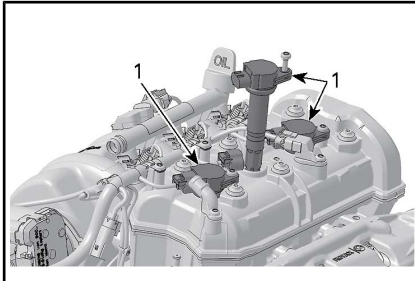
1. Zündspulen
