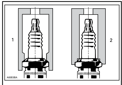
1. Geeigneter Steckschlüssel
