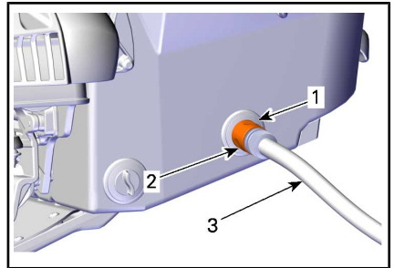
TYPISCH - SCHNELLKUPPLUNG
