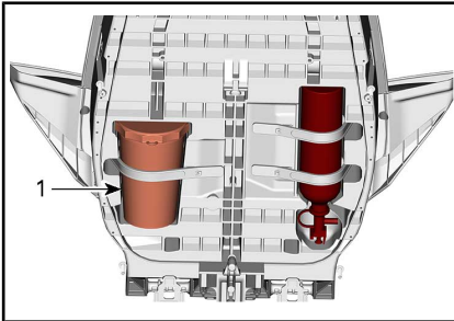
1. Sicherheitspaket
