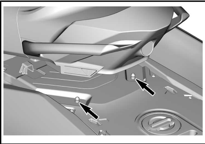
RASTSTIFTE
