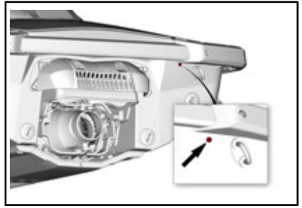
CONEXÃO DE TRANSBORDAMENTO DO INTERCOOLER
