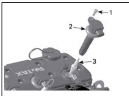
CONFIGURAZIONE TIPICA - TUTTI I MODELLI AD ECCEZIONE DEL 260 E DEI VEICOLI CON SISTEMA DI AMMORTIZZAZIONE
