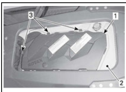
CONFIGURAZIONE TIPICA - MOTORI 260
