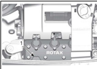
CONFIGURAZIONE TIPICA - TUTTI I MODELLI AD ECCEZIONE DEI MOTORI 260
