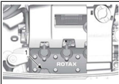
典型示例 - 260 发动机之外的所有型号
