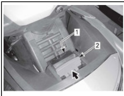
转向柱调整锁栓正确固定
