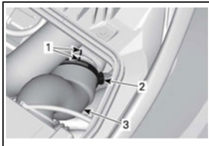
典型示例 - 1630 ACE HO 发动机
