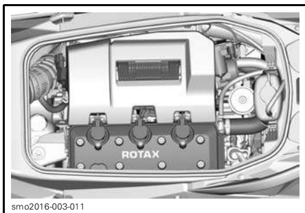
COMPARTIMENT MOTEUR, SIÈGE ENLEVÉ
