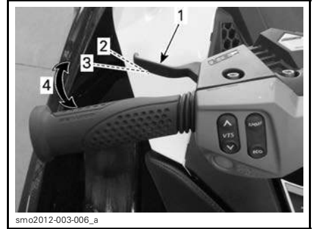
TIPIQUE - LEVIER iBR
