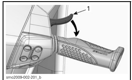
TYPBILD - LÄGGA I NEUTRAL 1. Gasreglage
