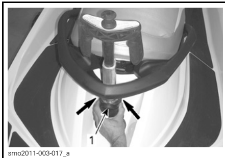
smo2011-003-017_a TYPBILD - TRYCK FRAMÅT FÖR ATT LÅSA UPP OCH TA BORT VATTENSKIDSTÅNGEN 1. Låsklämma
