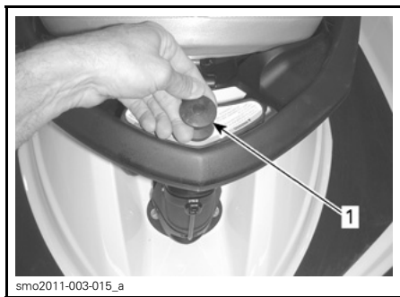
smo2011-003-015_a TYPBILD - NEDTRYCKT SKID-/WAKEBOARDSTÅNG 1. Dra i den här knoppen för att dra upp
