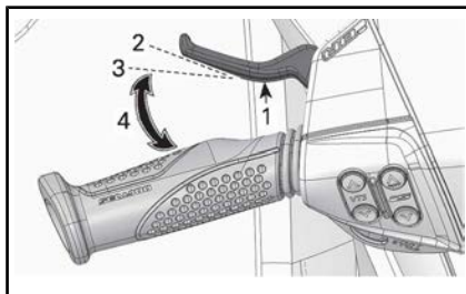
TÍPICO - PALANCA iBR
