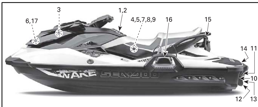
UBICACIÓN DE LAS ETIQUETAS DE SEGURIDAD EN LA MOTO ACUÁTICA - MODELOS WAKE
