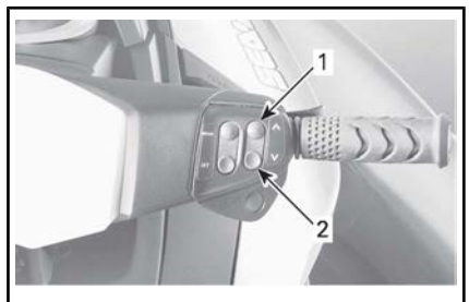
TÍPICO - AJUSTE DE LA POSICIÓN NEUTRA DE iBR
