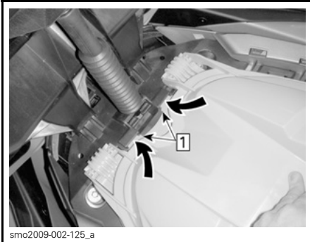
Step 1: Voorste lipjes van de opbergbak insteken
