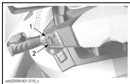
TYPISCH - VTS-REGELKNOP
