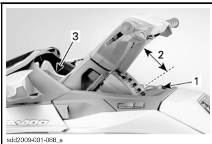
sdd2009-001-088_a TYPISCH 1. Klemmhebel 2. Mögliche Höheneinstellung 3. Multifunktionsanzeiginstrument
