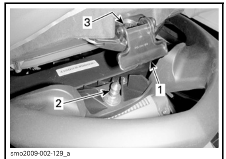
TYPISCH - SCHLIEßMECHANISMUS DES SITZES
