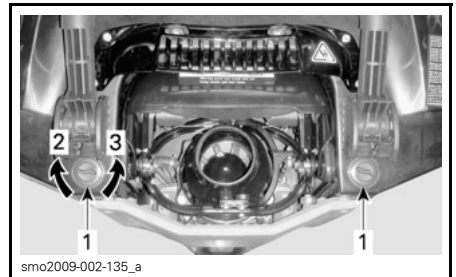
TYPISCH - LAGE DER BILGENABLAUFSTOPFEN
