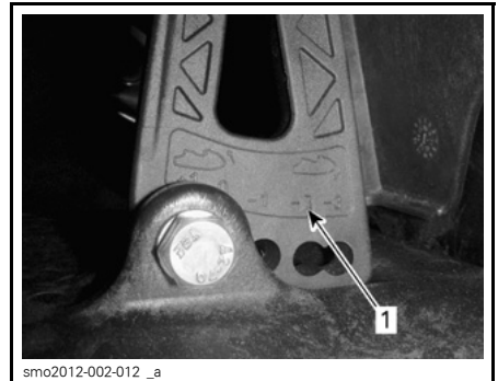
1. -Stellungen der Trimmungsklappe
