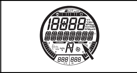
SPORT-MODUS-ANZEIGE (ALLE MODELLE AUSSER RXT-X/RXT-X aS)
