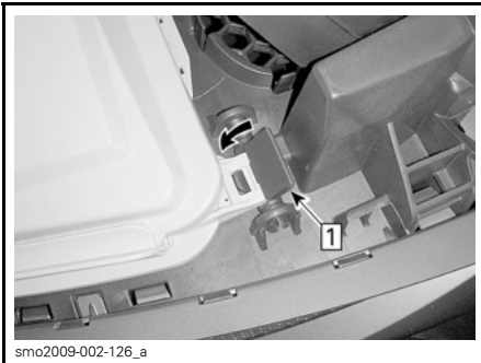
Schritt 1: Zum Sichern auf die Verriegelungen drücken
