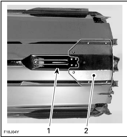
TYPIQUE — INSPECTER À CES ENDRITS 1. Admission d'eau 2. Plaque de promenade
