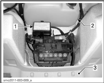
TYPIQUE 1. Boîte à fusibles 2. Réservoir d'essence 3. Compartiment de rangement avant (panneau d'accès retiré)
