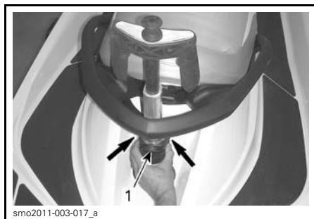
TYPIQUE - POUSSER VERS L'AVANT POUR DÉVERROUILLER ET ENLEVER LE POTEAU 1. Goupille de verrouillage
