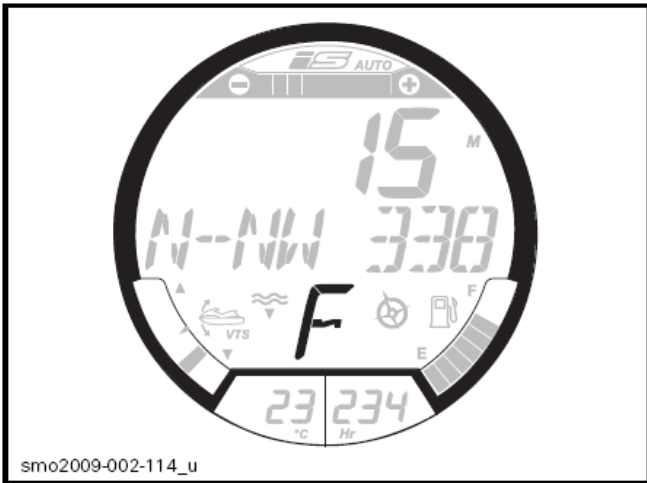
iBR 位置指示符
