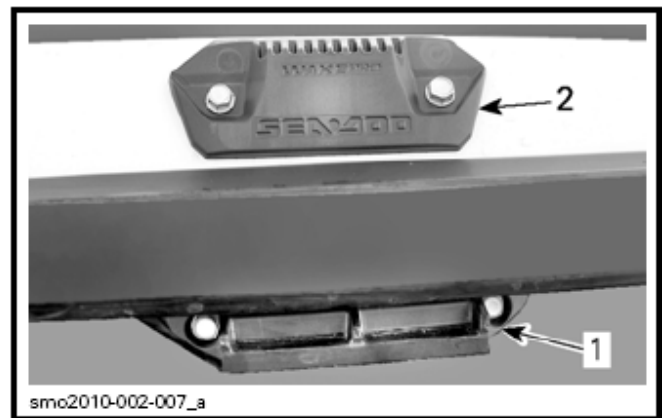
尾波板架的固定支架
