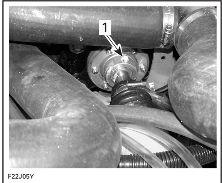
1. Smeer pakkinghouder van middenlager
