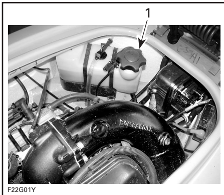
1. Dop olie-injectiereservoir
