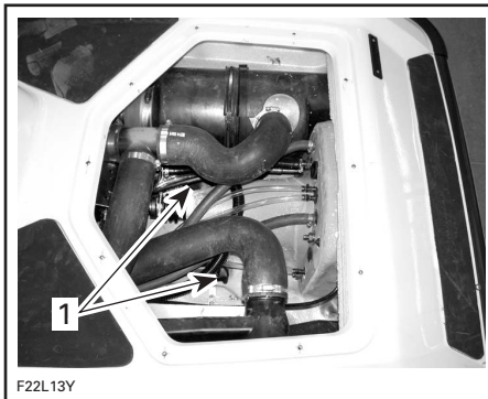
1. Aanzuigopeningen vacuüm-hoosysteem
