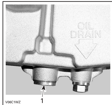
1. Oliezeefplug
