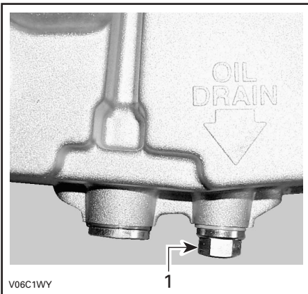
1. Olieaftapplug
