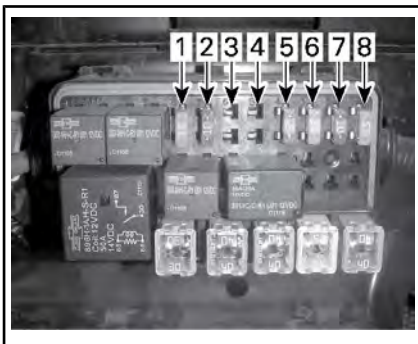
ПРЕДОХРАНИТЕЛИ — ЛЕВЫЙ БЛОК ПРЕДОХРАНИТЕЛЕЙ
