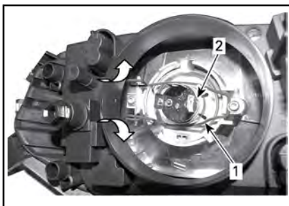
1. Пружинный фиксатор лампы
