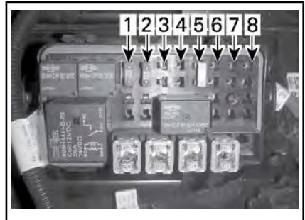
ПРЕДОХРАНИТЕЛИ — ПРАВЫЙ БЛОК ПРЕДОХРАНИТЕЛЕЙ
