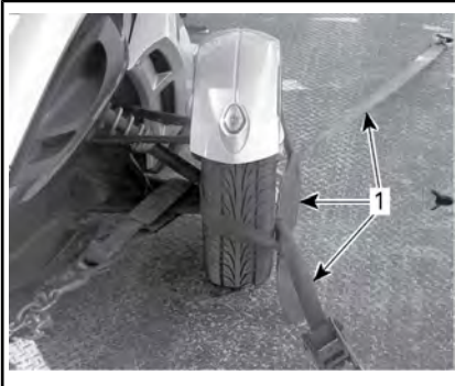
КРЕПЛЕНИЕ ПЕРЕДНИХ КОЛЕС — ТИПОВОЙ
