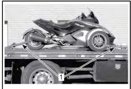
ТИПОВОЙ ВАРИАНТ — ТРАНСПОРТНОЕ СРЕДСТВО РАЗВЕРНУТО ПО ХОДУ БУКСИРОВКИ
