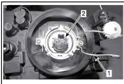
1. Пружинный фиксатор лампы
