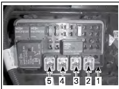
ПРЕДОХРАНИТЕЛИ В ИНДИВИДУАЛЬНОМ КОРПУСЕ — ПРАВЫЙ БЛОК ПРЕДОХРАНИТЕЛЕЙ
