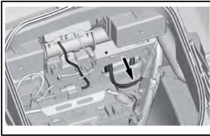
dc12 — ЦЕПЬ ДЛЯ ПОДКЛЮЧЕНИЯ ДОПОЛНИТЕЛЬНОГО ОБОРУДОВАНИЯ В ПЕРЕДНЕЙ ЧАСТИ — ЗА БАГАЖНЫМ ОТСЕКОМ
