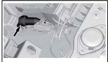
dc56 — ЦЕПЬ ДЛЯ ПОДКЛЮЧЕНИЯ ДОПОЛНИТЕЛЬНОГО ОБОРУДОВАНИЯ В ЗАДНЕЙ ЧАСТИ — ПОД СИДЕНЬЕМ ПАССАЖИРА
