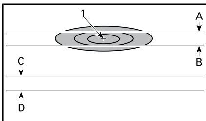
ТИПОВОЙ ВАРИАНТ — СВЕТ ФАРЫ НА ПРОВЕРОЧНОЙ ПОВЕРХНОСТИ — ДАЛЬНИЙ СВЕТ (ОДНА ФАРА)
