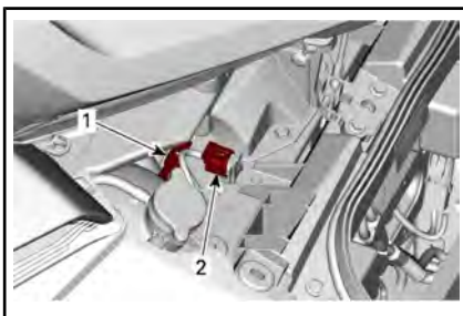
1. Диагностический разъем (для BUDS2) 2. 6-контактный разъем OBD2
