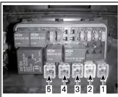
ПРЕДОХРАНИТЕЛИ В ИНДИВИДУАЛЬНОМ КОРПУСЕ — ЛЕВЫЙ БЛОК ПРЕДОХРАНИТЕЛЕЙ
