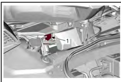
1. Диагностический разъем (для BUDS2)
