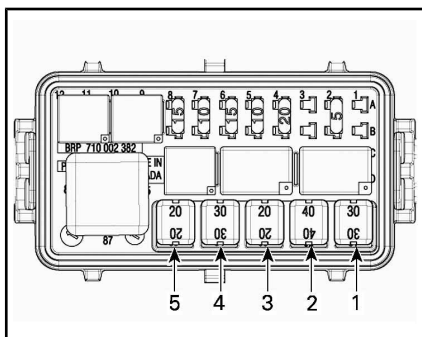
FUSIBLES HEMBRA: CAJA DE FUSIBLES DERECHA
