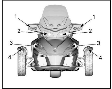
UBICACIÓN NORMAL DE LAS LUCES: PARTE DELANTERA DEL VEHÍCULO (TODOS LOS MODELOS EXCEPTO LOS MODELOS EUROPEOS)
