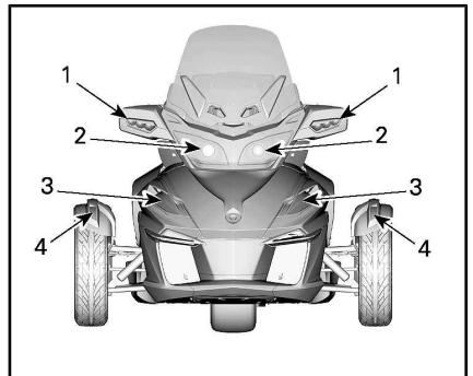
UBICACIÓN NORMAL DE LAS LUCES: PARTE DELANTERA DEL VEHÍCULO (MODELOS EUROPEOS)
