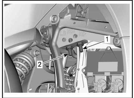
VISTA DE LA PARTE IZQUIERDA (MODELOS EUROPEOS Y AUSTRALIANOS)
