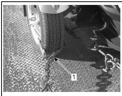
TÍPICO: FIJACIÓN DE LAS RUEDAS DELANTERAS — PRIMER MÉTODO
