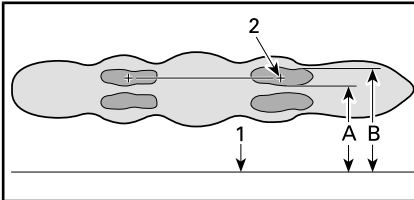
TÍPICO - REFLEJO DEL FARO EN LA SUPERFICIE DE PRUEBAS (AMBOS FAROS)
