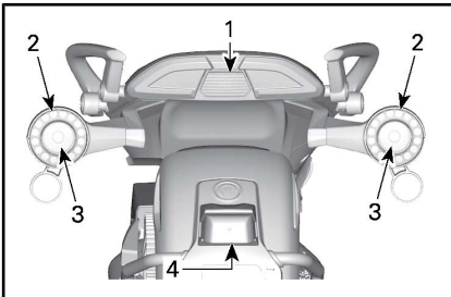
TÍPICO - LOCALIZAÇÃO DAS LUZS — TRASEIRA DO VEÍCULO — MODELOS F3 BASE E F3-S JAPONESES
