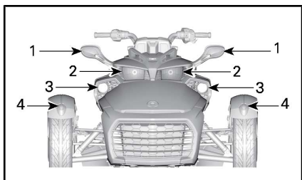
TÍPICO - LOCALIZAÇÃO DAS LUZES — FRENTE DO VEÍCULO - MODELOS PARA A AMÉRICA DO NORTE F3 BASE E F3-S
