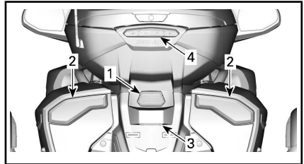
TÍPICO - LOCALIZAÇÃO DAS LUZS — TRASEIRA DO VEÍCULO — MODELOS F3 LIMITED - TODOS OS PAÍSES
