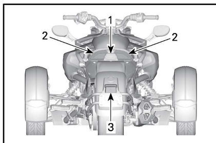
TÍPICO - LOCALIZAÇÃO DAS LUZES — TRASEIRA DO VEÍCULO - MODELOS F3 BASE E F3-S NORTE-AMERICANOS
