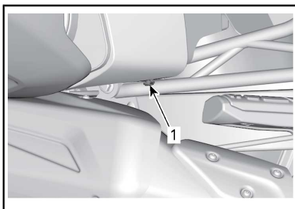
1. Rebite de plástico sob a parte frontal do alforje.
