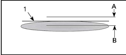
TÍPICO - PROJEÇÃO DO FAROL DIANTEIRO SOBRE A SUPERFÍCIE DE TESTE (UM FAROL)
