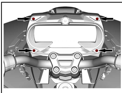
PARAFUSOS DE RETENÇÃO PARA REMOVER
