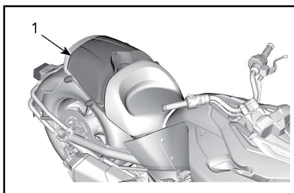
TÍPICO - LEVANTANDO O ASSENTO DO PASSAGEIRO PARA REMOVÊ-LO
