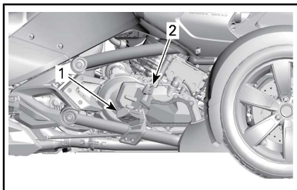
1. Botão do freio de estacionamento
