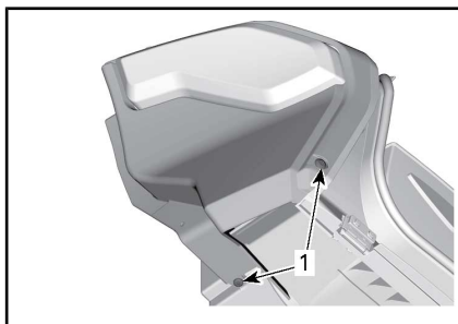
1. Parafusos de retenção inferiores para remover
