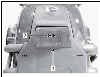
1. Parafusos de retenção inferiores para remover
