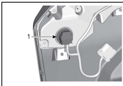
1. Gire o suporte da lâmpada para soltá-la.
