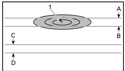
TÍPICO - PROJEÇÃO DO FAROL DIANTEIRO SOBRE A SUPERFÍCIE DE TESTE — FAROL ALTO (UM FAROL)
