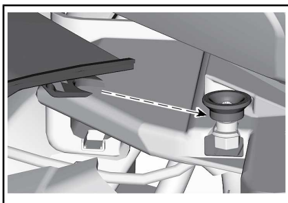
TÍPICO - ALINHAMENTO DE ABAS NO LOCAL CORRETO DE INSTALAÇÃO
