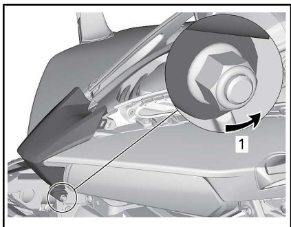
TÍPICO - NARIZ DO CONSOLE PIVOTEANDO
