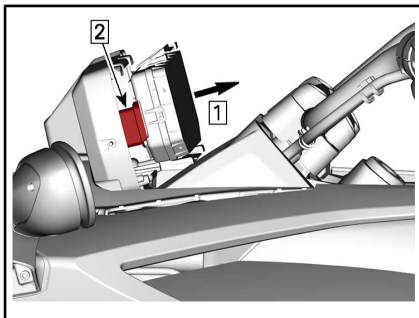
Passo 1: Remover o indicador Passo 2: desconectar
