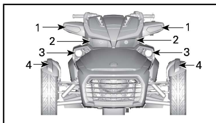
TÍPICO - LOCALIZAÇÃO DAS LUZES — FRENTE DO VEÍCULO - MODELOS F3-T E F3 LIMITED EUROPEUS, AUSTRALIANOS E JAPONESES
