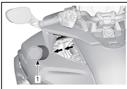
TÍPICO - REMOÇÃO DO FILTRO DE AR DO SILENCIADOR DA ADMISSÃO DE AR.
