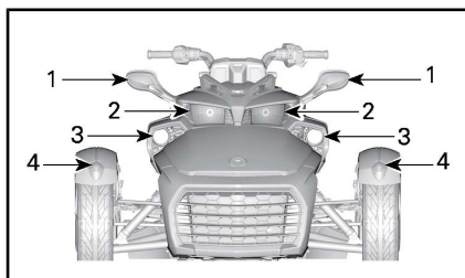
TÍPICO - LOCALIZAÇÃO DAS LUZES — FRENTE DO VEÍCULO — MODELOS F3 BASE E F3-S EUROPEUS, AUSTRALIANOS E JAPONESES
