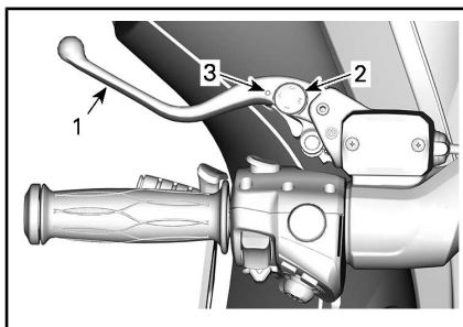
TÍPICO - AJUSTE DA ALAVANCA DA EMBREAGEM
