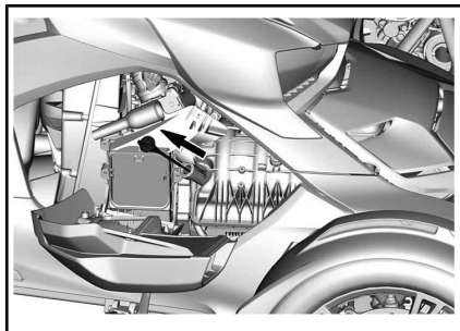
MOTORE 900 ACE
