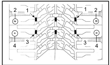
ILLUSTRAZIONE PNEUMATICO POSTERIORE
