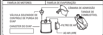
TÍPICO - LOCALIZAÇÃO DE ETIQUETAS DE CONFORMIDADE
