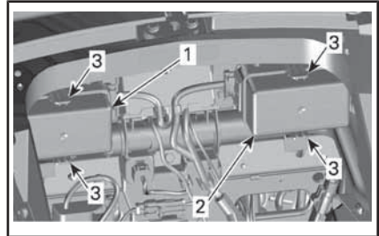
DENTRO DO BAGAGEIRO DIANTEIRO
