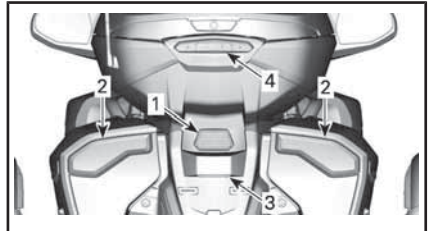
TÍPICO - LOCALIZAÇÃO DAS LUZES — TRASEIRA DO VEÍCULO — MODELOS F3 LIMITED - TODOS OS PAÍSES
