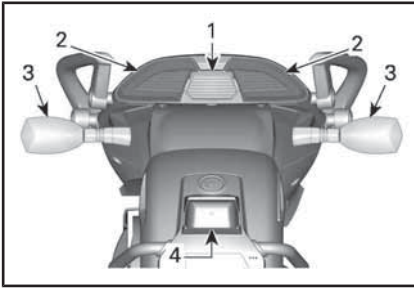
TÍPICO - LOCALIZAÇÃO DA LUZES — TRASEIRA DO VEÍCULO - TODOS OS MODELOS, EXCETO OS MODELOS F3 LIMITED E F3-T NORTE-AMERICANOS E JAPONESES
