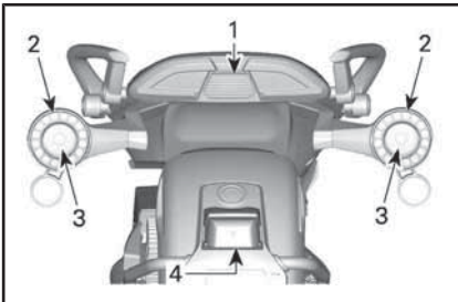
TÍPICO - LOCALIZAÇÃO DAS LUZES — TRASEIRA DO VEÍCULO — MODELOS F3 BASE E F3-S JAPONESES
