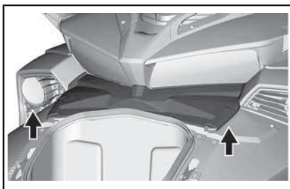
TÍPICO - LEVANTAMENTO DA TAMPA DE MANUTENÇÃO
