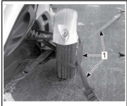
TÍPICO - SUJECIÓN DE LAS RUEDAS DELANTERAS
