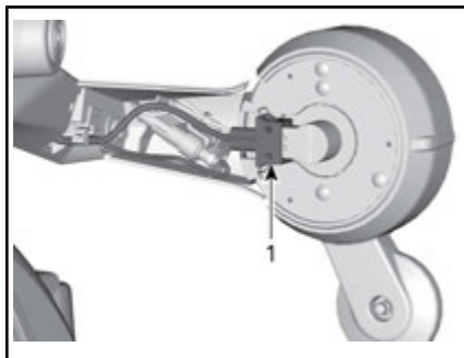
1. Desconecte el conector del intermitente
