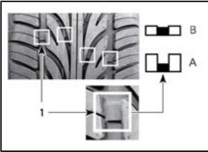
DESGASTE DE LA BANDA DE RODADURA
