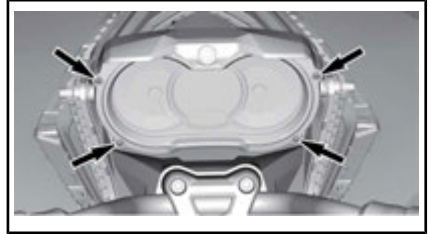
TORNILLOS DE SUJECIÓN QUE DEBEN QUITARSE
