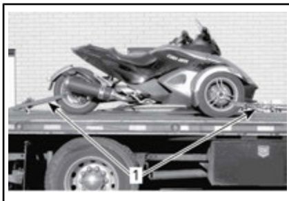
TÍPICO - VEHÍCULO ORIENTADO HACIA EL REMOLQUE
