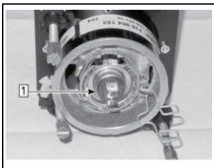
Etap 1: Extraiga la lámpara del alojamiento
