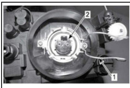
1. Muelle de retención de la lámpara
