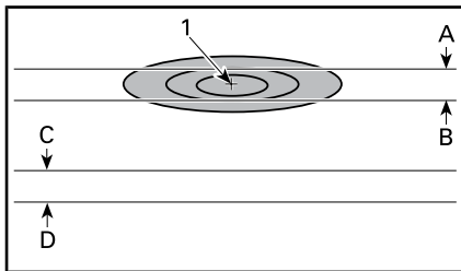
TÍPICO - REFLEJO DEL FARO SOBRE LA SUPERFICIE DE PRUEBAS - LUZ LARGA (UN SOLO FARO)
