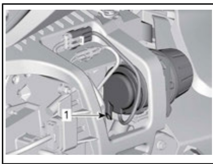
1. Tubo del respiradero orientado hacia abajo
