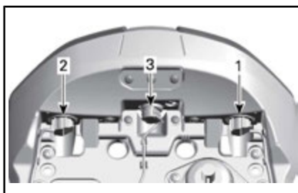
1. Desconecte el conector del intermitente
