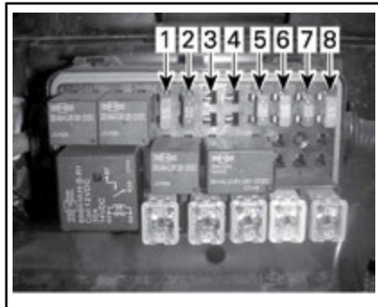
FUSIBLES: CAJA DE FUSIBLES IZQUIERDA
