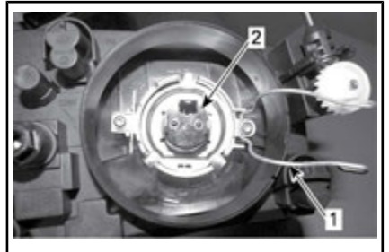
1. Muelle de retención de la lámpara
