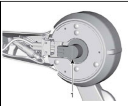
1. Gire el portalámparas para liberarlo.
