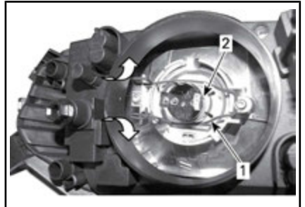
1. Muelle de retención de la lámpara
