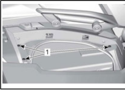
1. Tornillos de sujeción que deben quitarse
