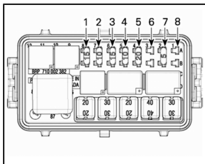
SULAKKEET – OIKEA SULAKEKOTELO
