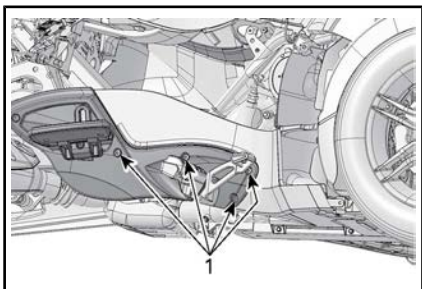
1. Kiinnitysruuvit
