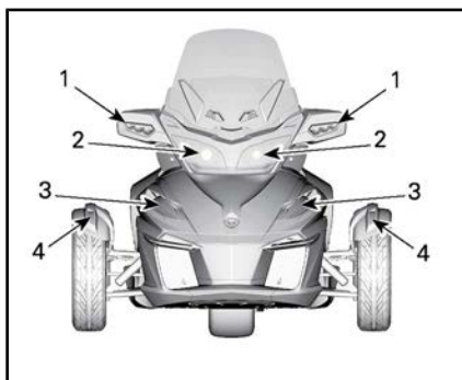
UBICACIÓN NORMAL DE LAS LUCES: PARTE DELANTERA DEL VEHÍCULO (MODELOS EUROPEOS)
